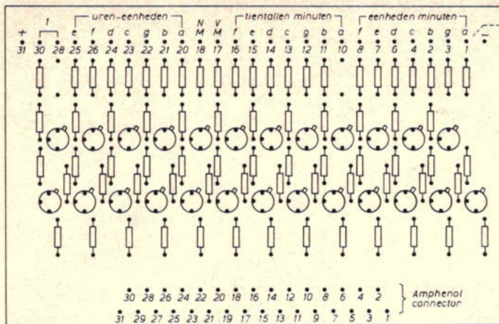
Fig. 5b. Componentenopstelling van de LED-stuurtrap.
